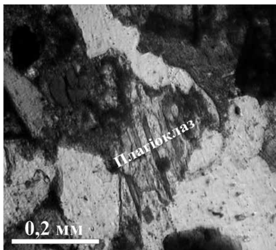
Рис. 8. Пісковик кварцово-глауконітовий, дрібнозернистий, алевритистий, із карбонатним цементом (свердловина Одеська-2, інт. 1189-1196 м, середній еоцен, нік. II)
