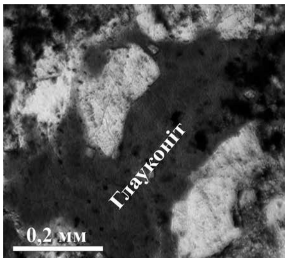
Рис. 9. Пісковик кварцово-глауконітовий, різнозернистий із карбонатно-глинистим цементом (свердловина Одеська-2, інт. 1205-1214 м, середній еоцен, нік. II)
