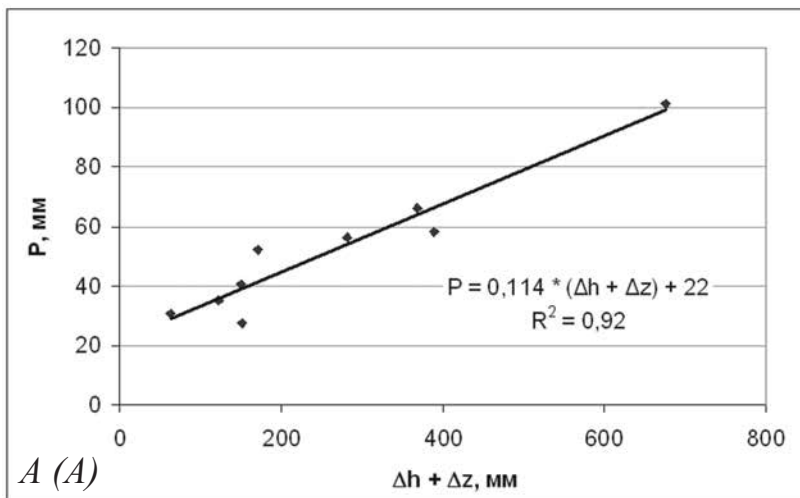
Рис. 2. Кореляційний аналіз залежностей між параметрами із застосуванням лінійної регресії
