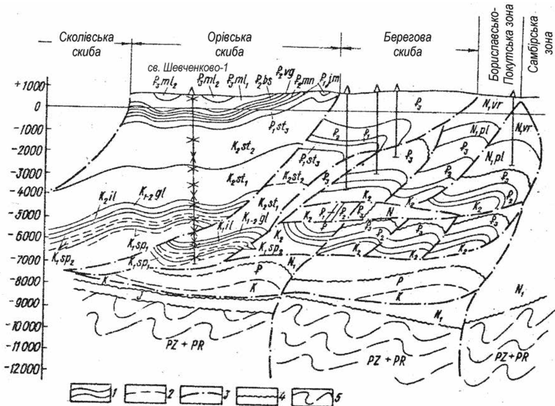
Рис. 1А. – Геологічний профіль району свердловини Шевченково-1: 1 – стратиграфічні межі світ і підсвіт; 2 – межі пачок; 3 – тектонічні порушення, надвиги; 4 – незгідне залягання порід; 5 – складчастий фундамент
