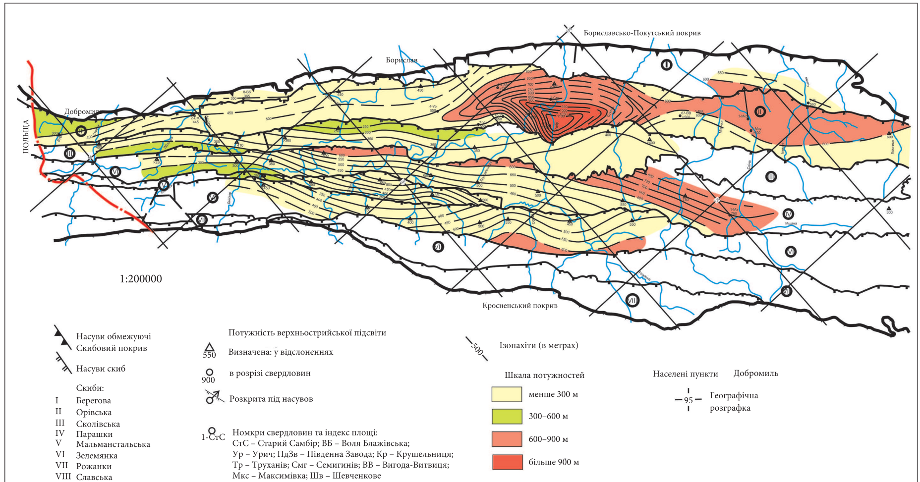
Рис. 3. Карта товщини верхньострийської підсвіти в північно-західній і центральній частинах Скибового покриву
