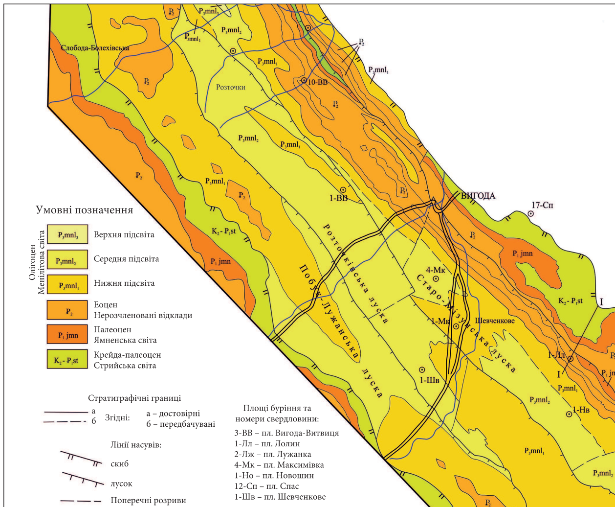
Рис. 6. Геологічна карта Скибового покриву в межиріччі Ілемка–Лужанка. Викопійована з модернізованої у 2019 р. карти В.В. Глушка, В.В. Кузовенка і В.Є. Шлапінського (2007 р.). Масштаб 1 : 100 000
