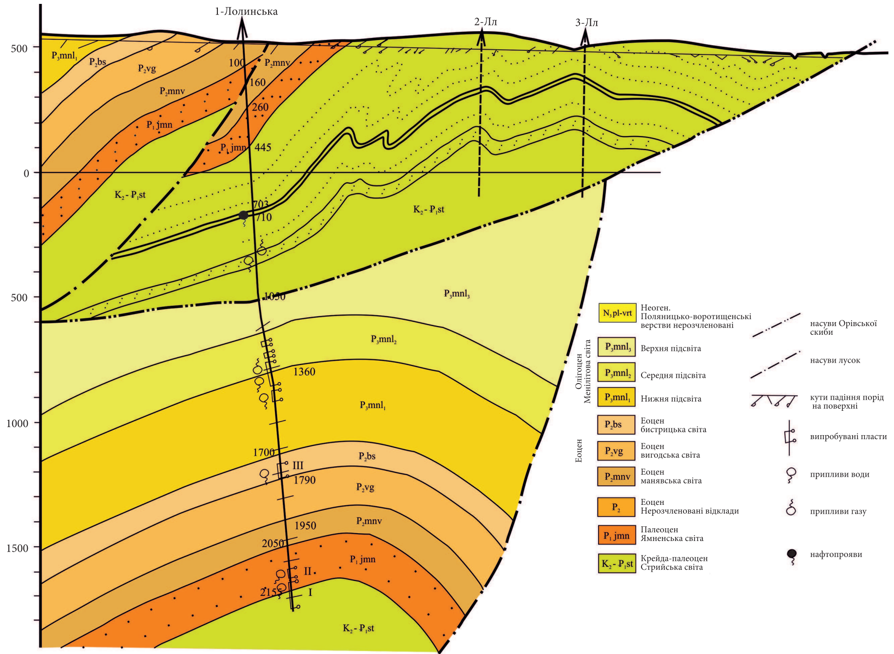
Рис. 5. Геологічний профіль через свердловину 1-Лолінська. Склад В.В. Кузовенко (2004 р.). Масштаб 1 : 10 000
