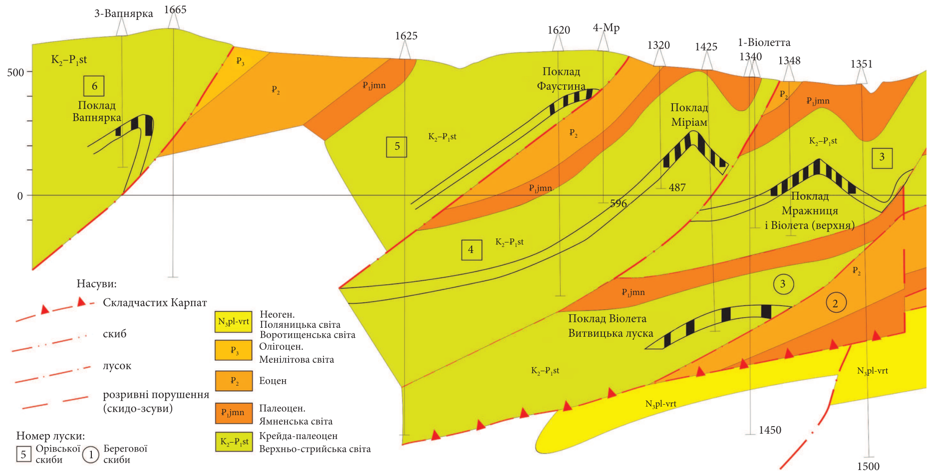
Рис. 4. Геологічний профіль по лінії свердловин 3-Вапнярка — 1351-Борислав (Мражницький перетин). Склад В.Є. Шлапінський у 2019 р.
