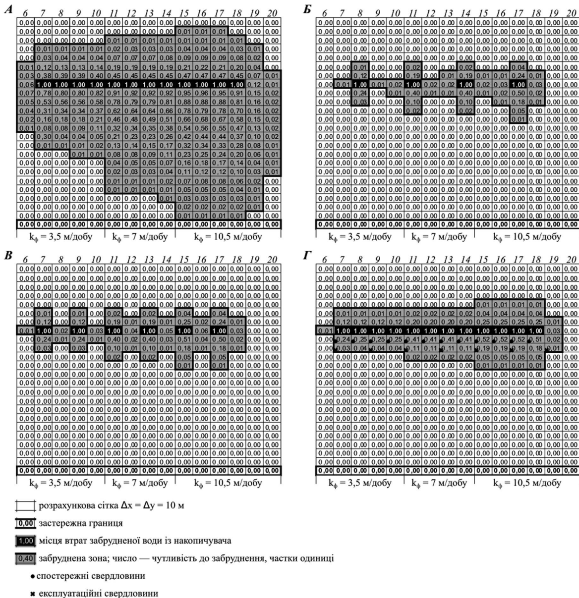
Рис. 2. Варіанти моделювання розповсюдження забруднювача: при суцільних втратах протягом 90 діб (А); протягом 10 діб при втратах із джерела забруднення через 20 м (Б); протягом 10 діб при втратах із джерела забруднення через 10 м (В); при суцільних втратах упродовж 10 діб (Г)
